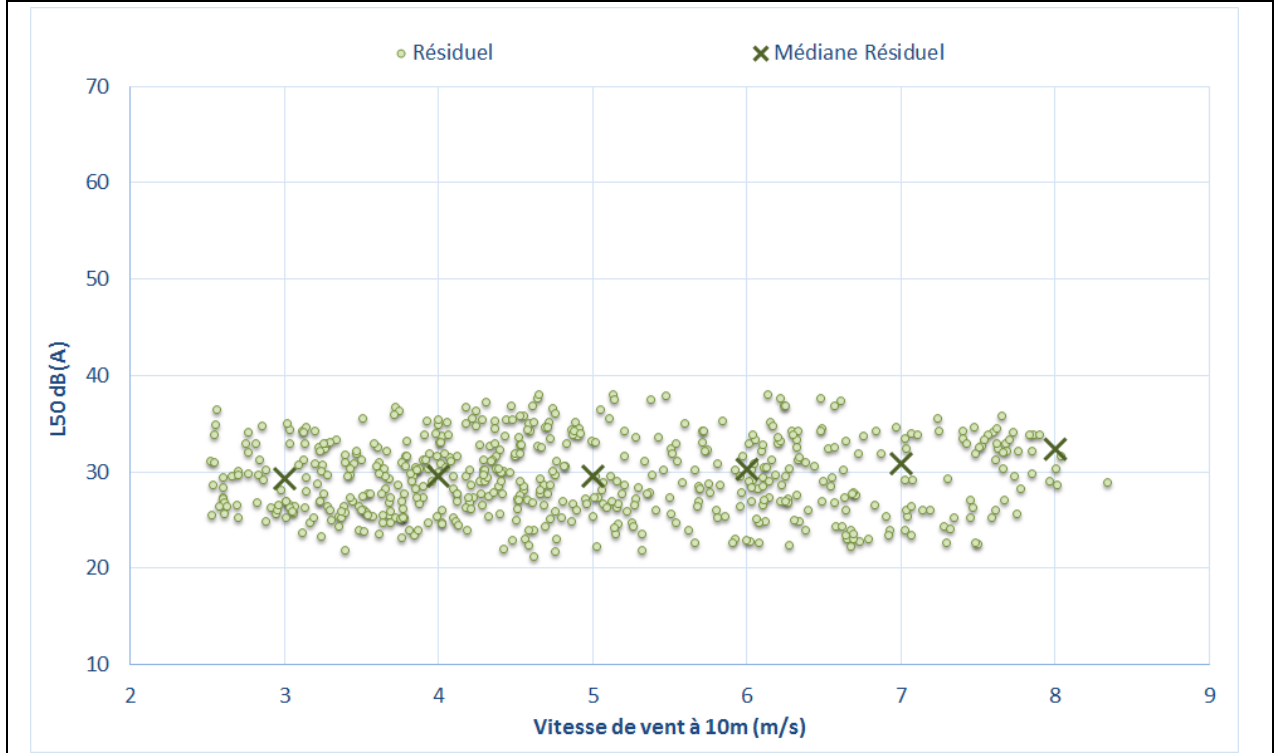
Figure 31 : Bruit en fonction de la vitesse de vent au point P10 – Mesures estivales
