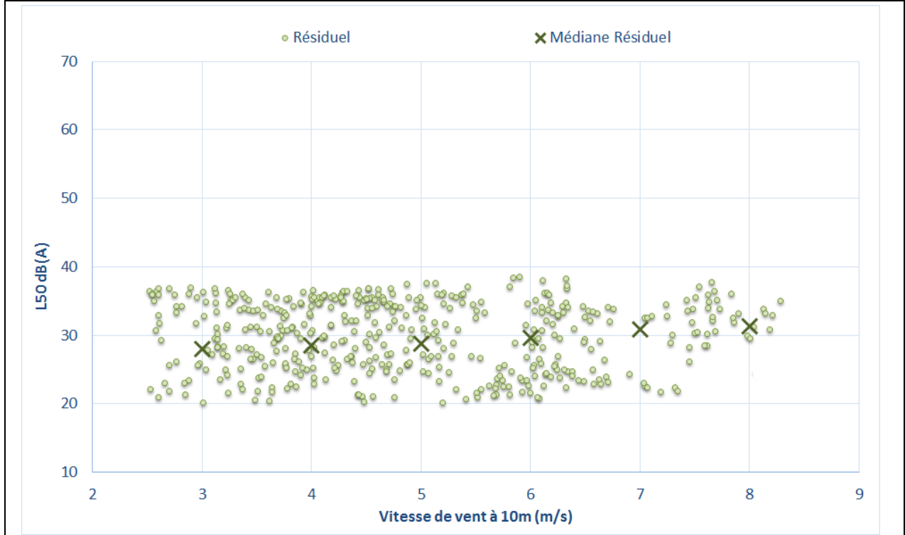
Figure 34 : Bruit en fonction de la vitesse de vent au point P13 – Mesures estivales
