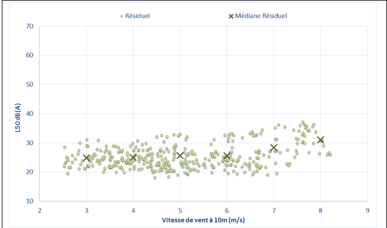
Figure 33 : Bruit en fonction de la vitesse de vent au point P12 – Mesures estivales
