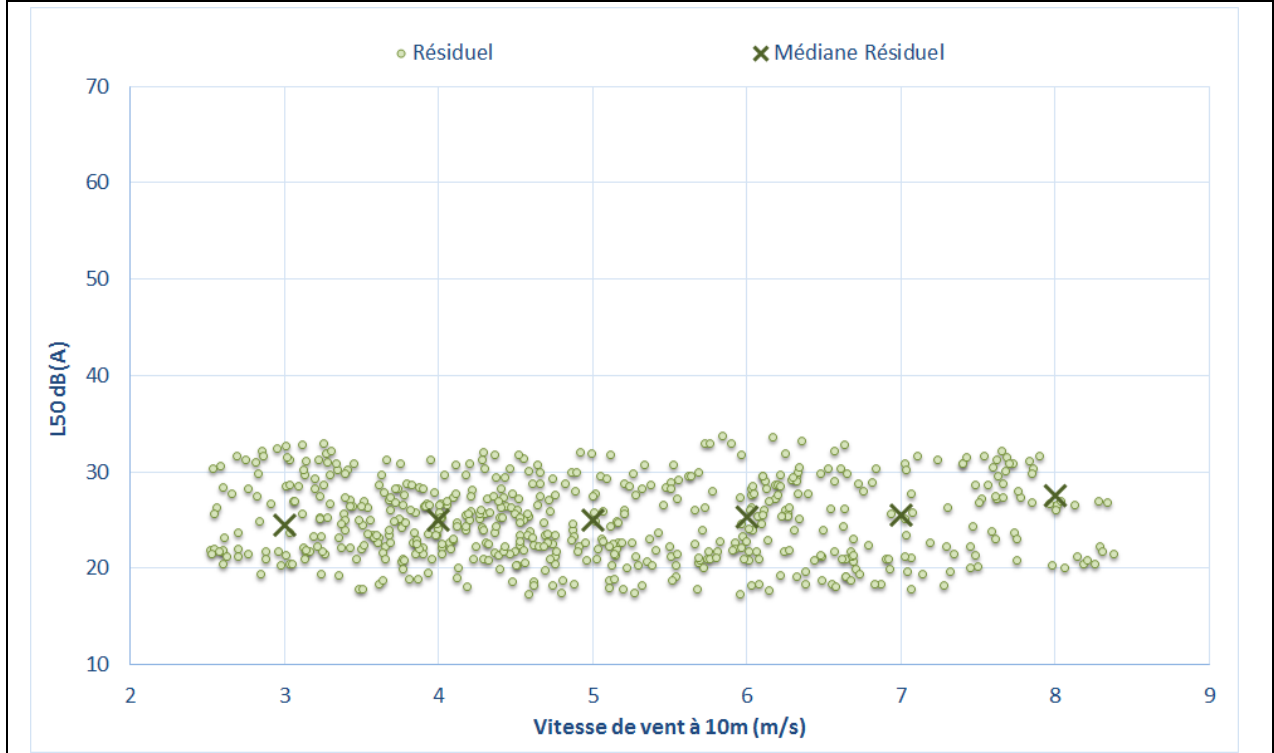
Figure 32 : Bruit en fonction de la vitesse de vent au point P11 – Mesures estivales
