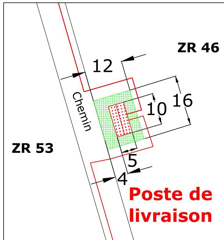
Plan de masse du poste de livraison
