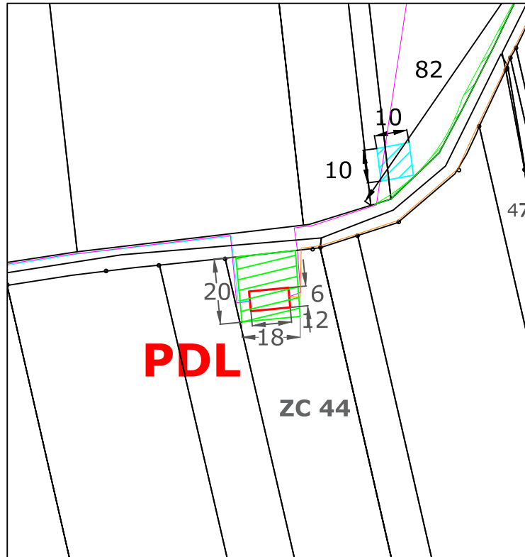
Plan de masse du poste de livraison 6 X 12 m
