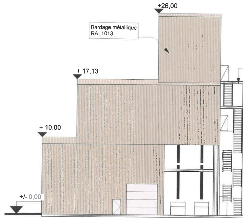
- Façade Sud - 1/250 -
