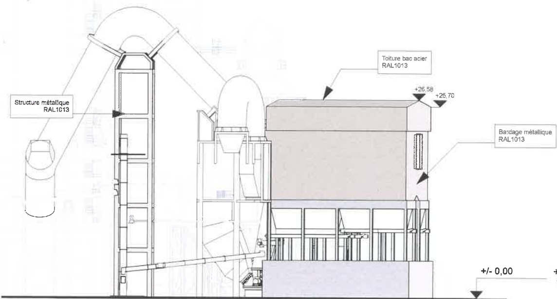
- Façade Ouest - 1/500 -
