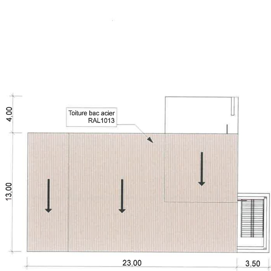
- Plan de toiture - 1/250 -
