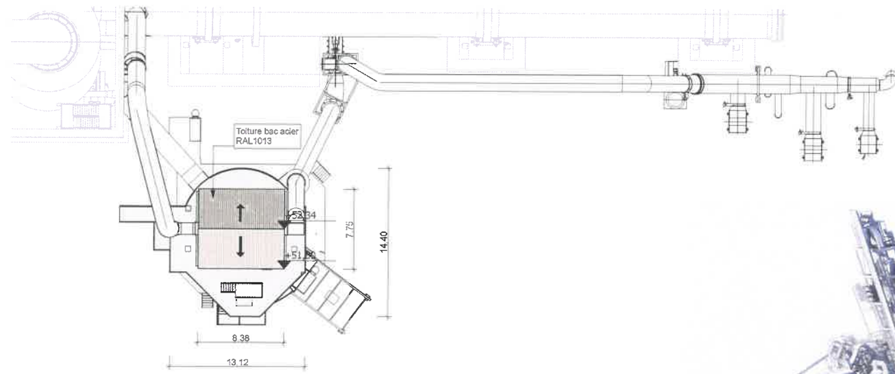
- Plan de toiture - 1/500 -
