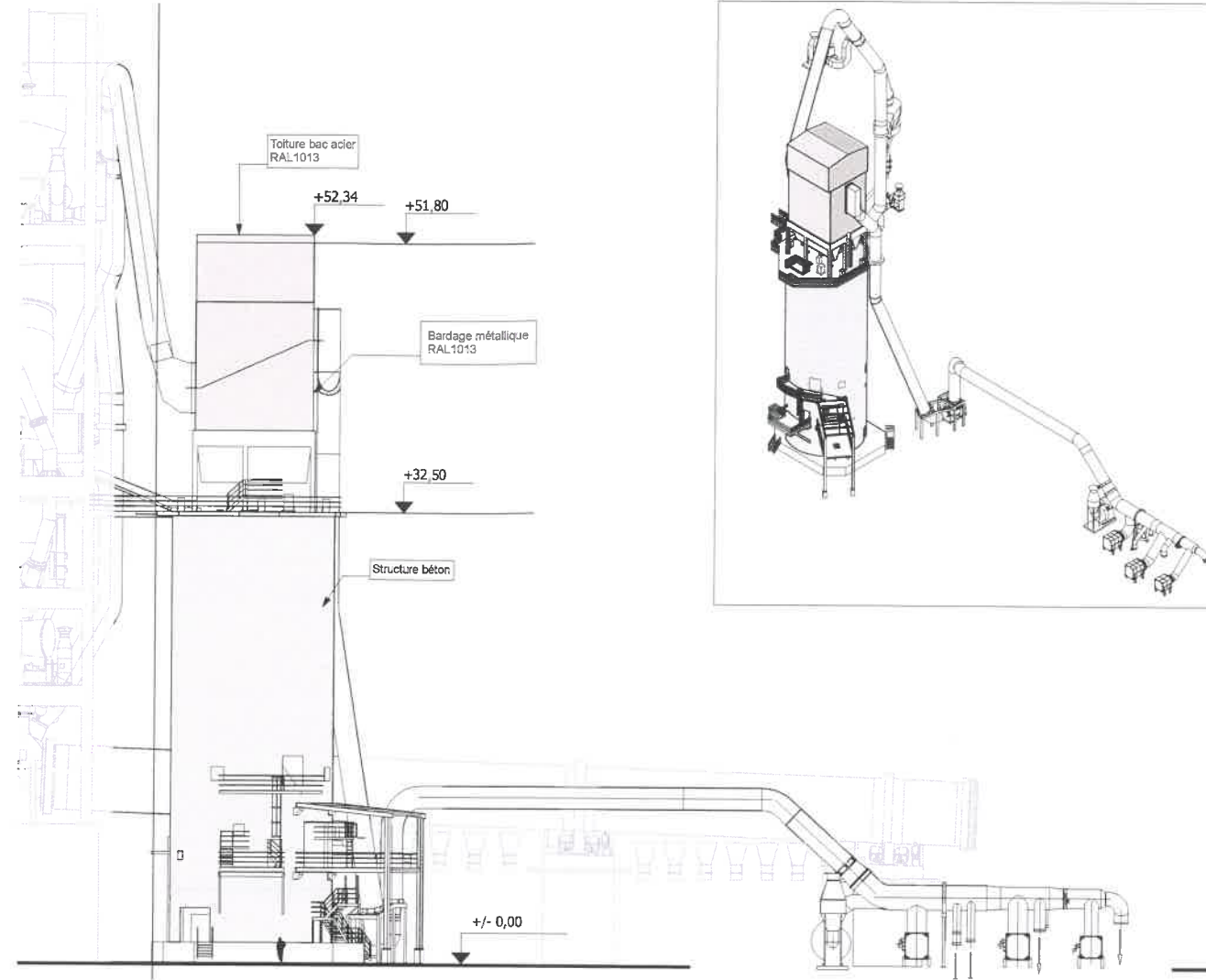
- Façade Sud - 1/500 -
