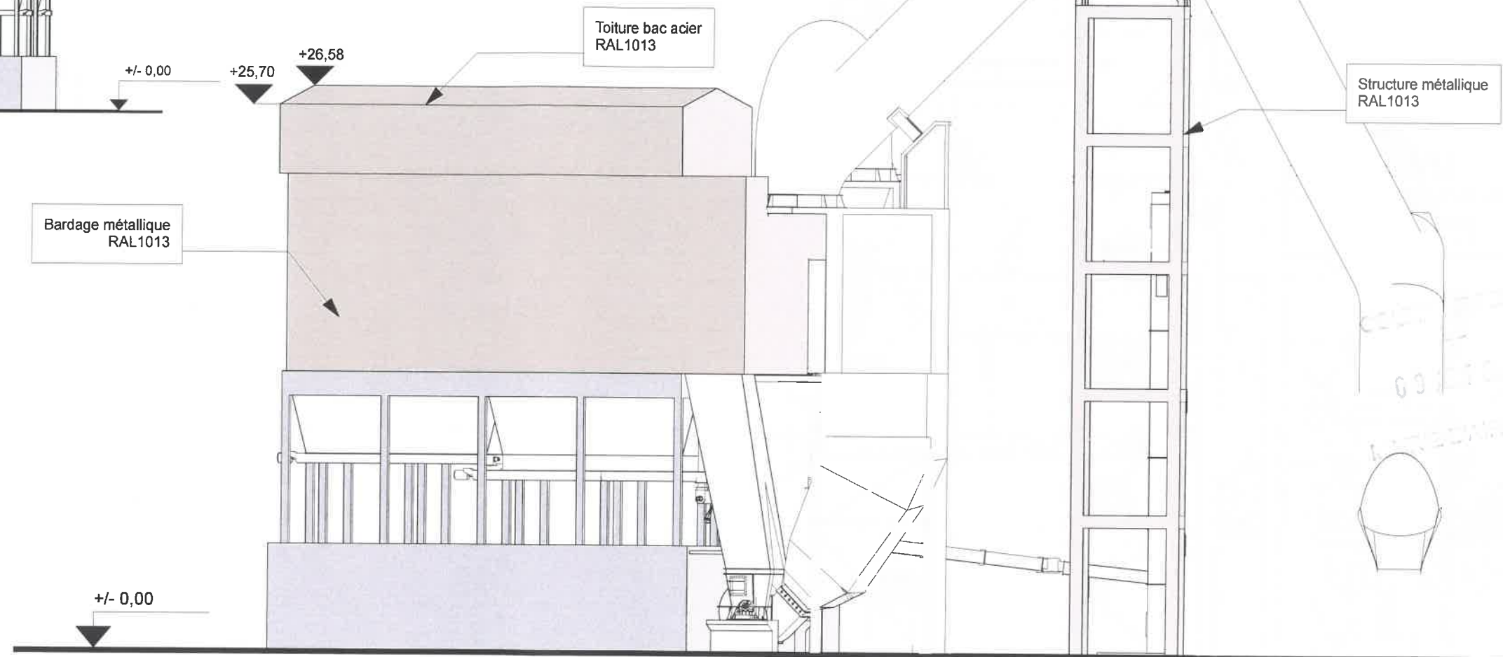
- Façade Est - 1/250 -
