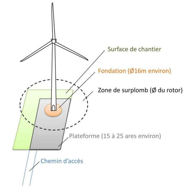
Illustration 2 : exemple d'emprises au sol d'une éolienne
