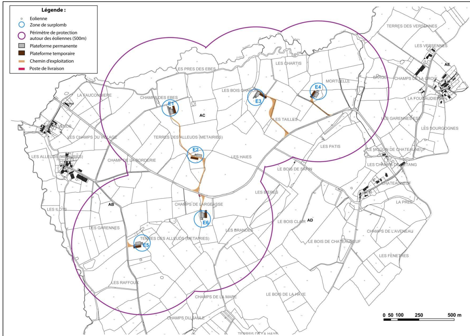
Carte 8 : plan masse de l'ensemble de l'installation
