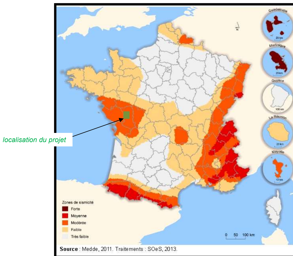
Carte 5 : Zonage de l'aléa sismique pour la France
