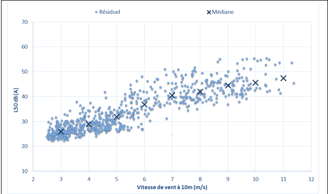
Figure 13 : Bruit en fonction de la vitesse de vent au point P9 – Mesures hivernales
