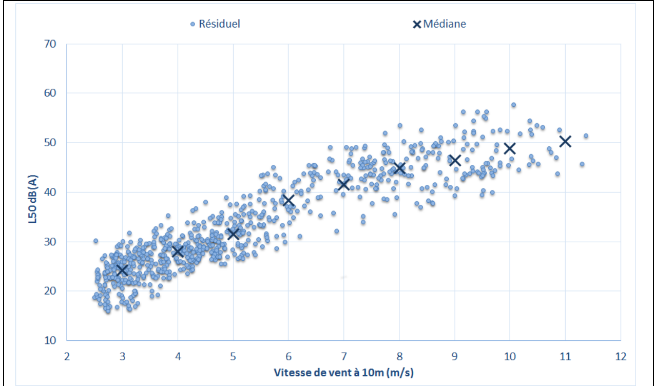
Figure 14 : Bruit en fonction de la vitesse de vent au point P10 – Mesures hivernales
