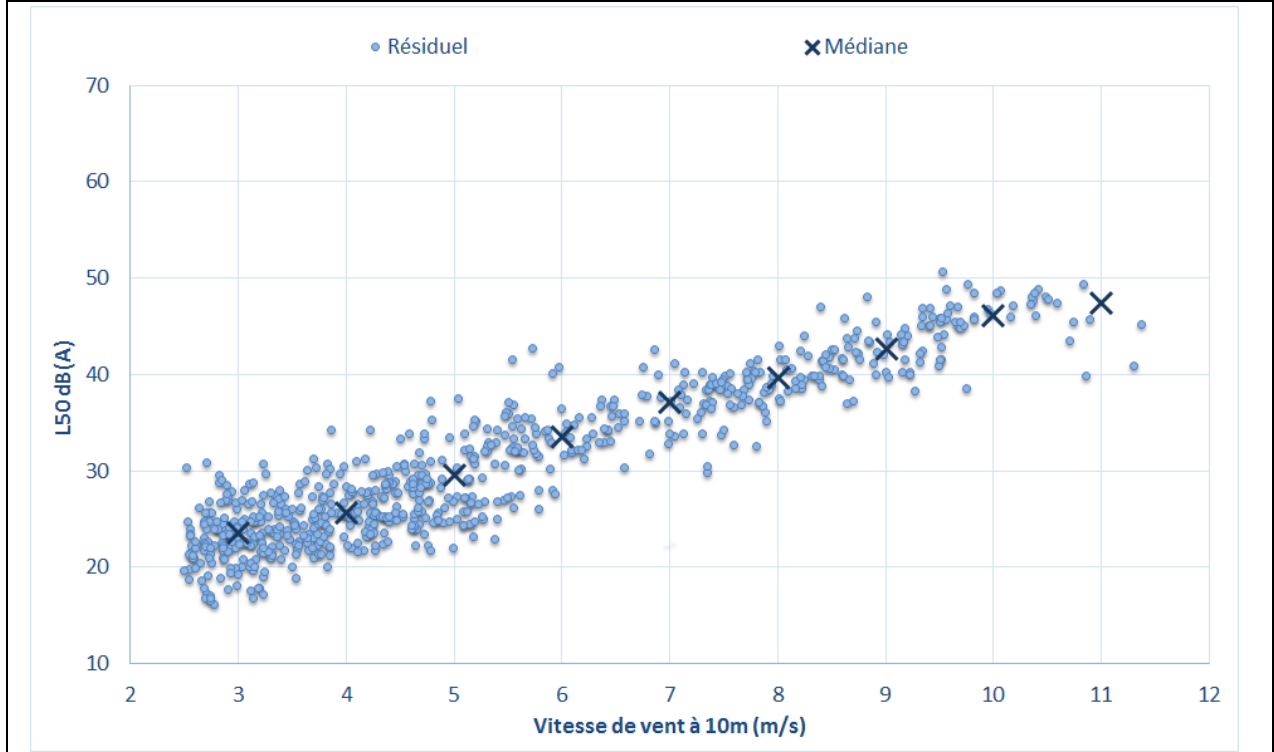
Figure 15 : Bruit en fonction de la vitesse de vent au point P11 – Mesures hivernales
