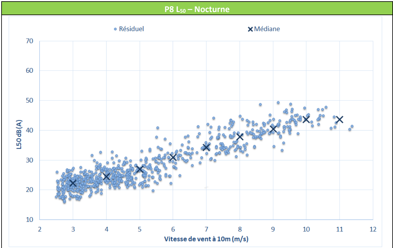
Figure 12 : Bruit en fonction de la vitesse de vent au point P8 – Mesures hivernales
